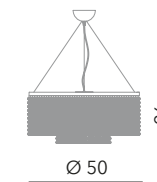
lampadario rotondo 6L Ø 50 cm - H 26 cm 6 x G9 60W
