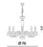
lampadario 8L Ø 76 cm - H 57 cm 8 x E14 40W
