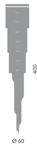
Mosca plafoniera Ø 60 cm Ø 60 cm - H 400 cm 20 x E14 40W
