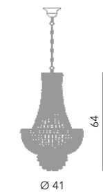
Roma lampadario Impero Ø 40 cm Ø 41 cm - H 64 cm 6 x E14 40W
