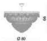
sospensione Ø 80 cm Ø 80 cm - H 66 cm 12 x E14 40W
