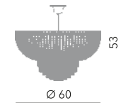
Monaco sospensione Ø 60 cm Ø 60 cm - H 53 cm 8 x E14 40W
