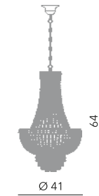
Monaco sospensione Ø 40 cm Ø 41 cm - H 64 cm 6 x E14 40W
