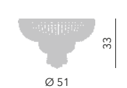
Asburgo plafoniera Ø 50 cm Ø 51 cm - H 33 cm 6 x E14 40W
