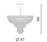
Asburgo sospensione Ø 40 cm Ø 41 cm - H 46 cm 4 x E14 40W
