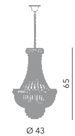
Borbone lampadario Impero Ø 40 cm Ø 43 cm - H 65 cm 6 x E14 40W
