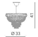
Borbone sospensione Ø 30 cm Ø 33 cm - H 41 cm 3 x E14 40W
