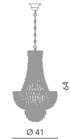
Stuart lampadario Impero Ø 40 cm Ø 41 cm - H 64 cm 6 x E14 40W
