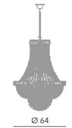
Borbone lampadario Impero Ø 60 cm Ø 64 cm - H 86 cm 9 x E14 40W
