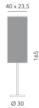
terra ovale 8L base Ø 30 - vetro 40 x 23,5 - H 165 cm 8 x G9 60W
