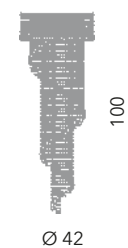
Mosca plafoniera Ø 40 cm Ø 42 cm - H 100 cm 12 x E14 40W
