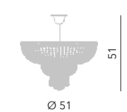
Asburgo sospensione Ø 50 cm Ø 51 cm - H 51 cm 6 x E14 40W
