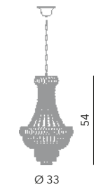
Borbone lampadario Impero Ø 30 cm Ø 33 cm - H 54 cm 5 x E14 40W
