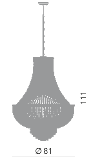
Stuart lampadario Impero Ø 80 cm Ø 81 cm - H 111 cm 15 x E14 40W
