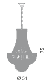
Roma lampadario Impero Ø 50 cm Ø 51 cm - H 75 cm 7 x E14 40W
