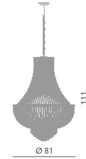
Monaco sospensione Ø 80 cm Ø 81 cm - H 111 cm 15 x E14 40W
