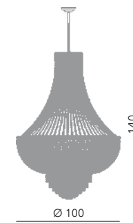
Roma lampadario Impero Ø 100 cm Ø 100 cm - H 140 cm 18 x E14 40W
